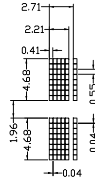
DETAIL:DOTS SCALE: 2:1
